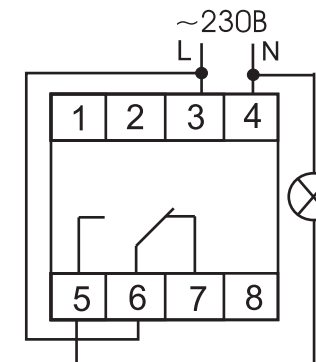
Рис.1 Рекомендуемая схема подключения таймера PCZ-521-1 и нагрузки к сети 230В.
