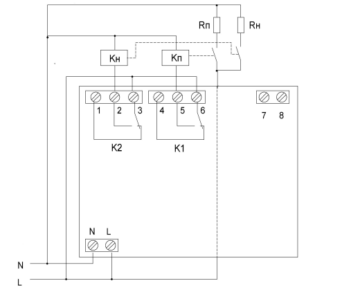
Kн, Kп-контакты с нормально разомкнутыми контактами
