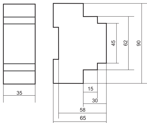
Рис. 5 Габаритные размеры.
