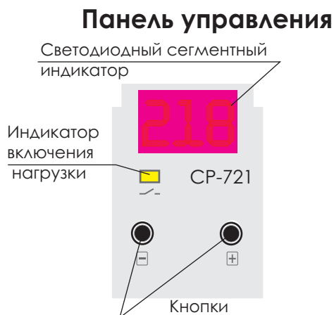
Рис.1 Расположение органов индикации и управления.
