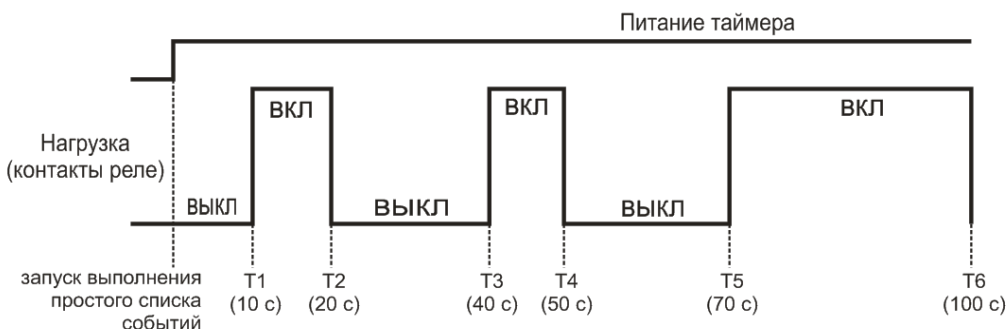
Рисунок 6.9 – Включение нагрузки на примере простого режима работы
