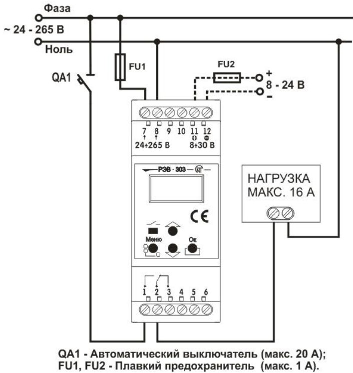
Рисунок 5.1 – Схема подключения РЭВ-303
