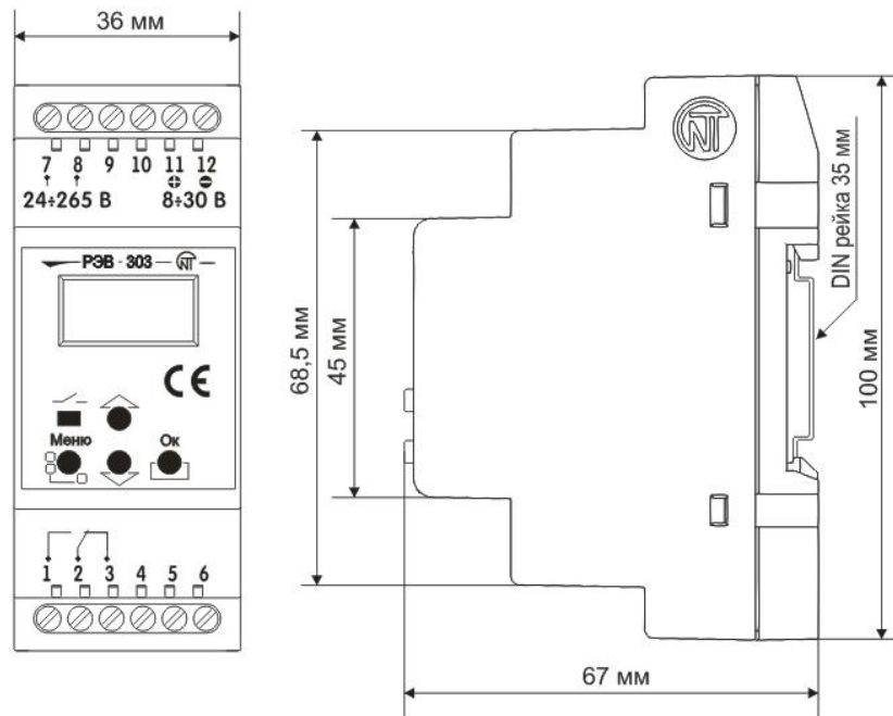
Рисунок 3.1 – Внешний вид и габаритные размеры таймера
