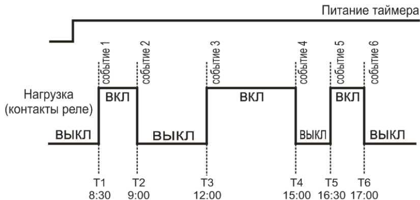
Рисунок 6.8 – Включение нагрузки на примере суточного режима работы
